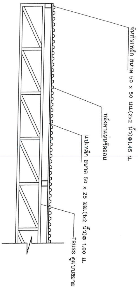
แบบขยาย โครงหลังคา Scale 1:50
